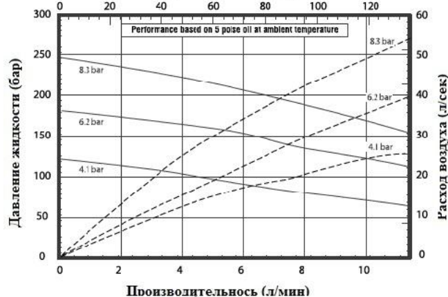
Кривые производительности Циклы в минуту
