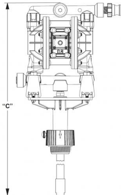
Габаритные размеры
