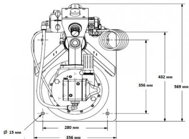
Габаритные и монтажные размеры
