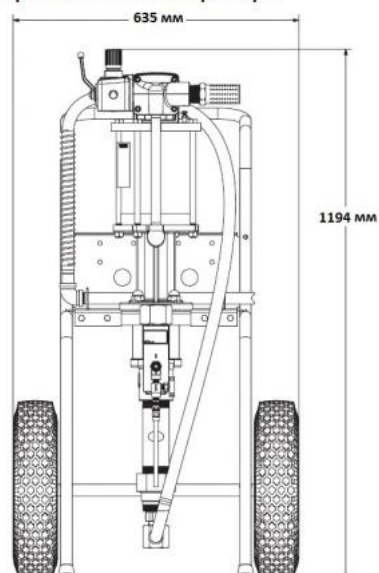
Габаритные и монтажные размеры
